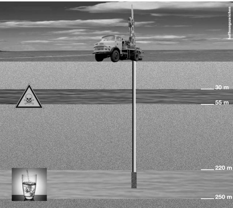
Das Bohrgerät in Bouw musste sehr tief bohren, um den unteren Wasserleiter zu erschließen. Der oberste Wasserleiter ist mit Chemie-Abfällen des Ölindustrie verschmutzt.
